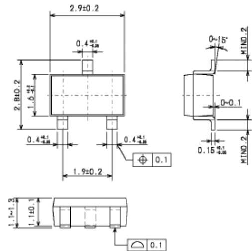
SOT23-3/SOT23-3B
