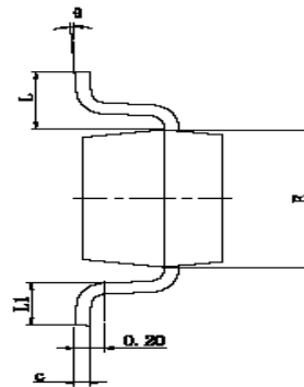
SOT353
